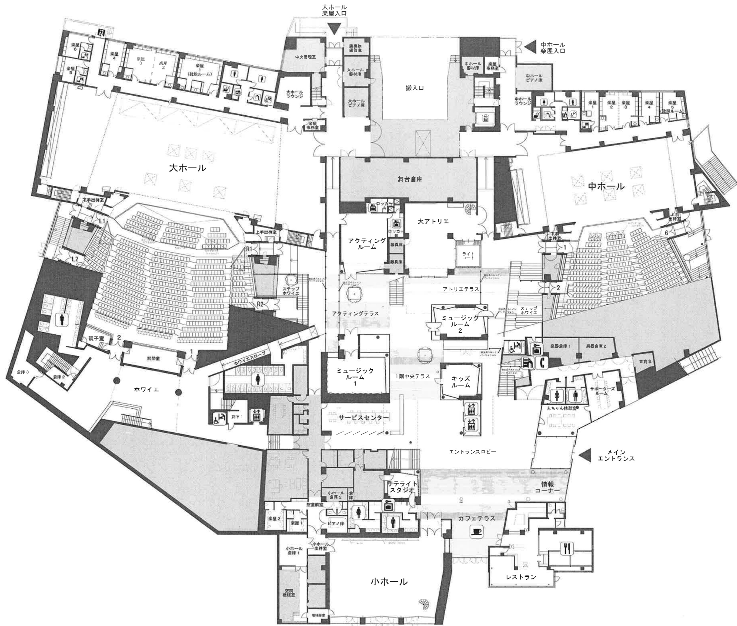
北上市文化交流センター さくらホール 1階 全体平面図 S = 1:400
