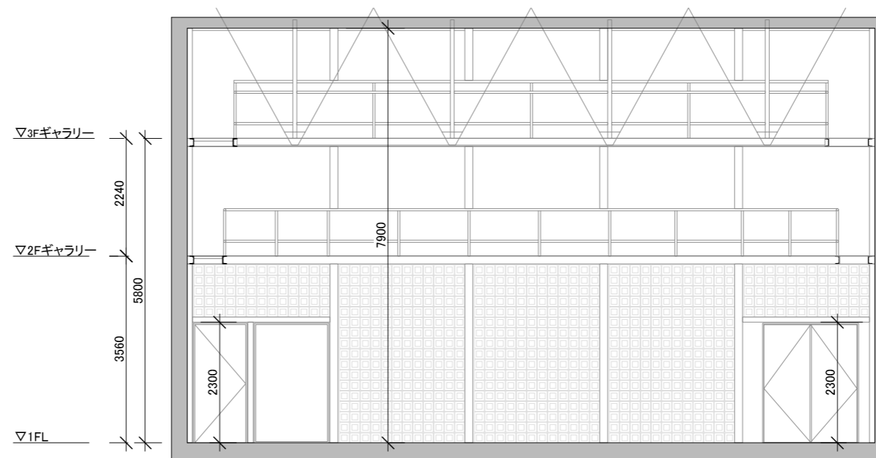
断面図 B-B'
