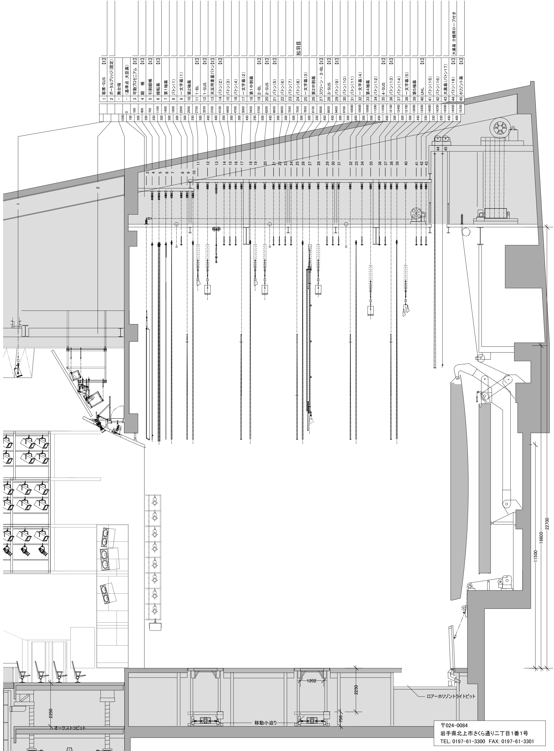
大ホール舞台断面図 S=1:100
